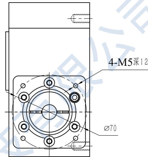
B视图
