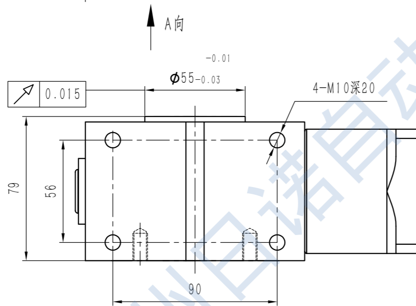
A视图
